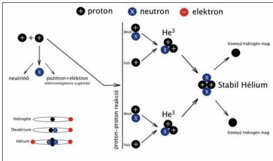
A proton-proton reakció folyamata, a Napunk esetében többségben így jön létre hélium, illetve keletkezik energia (ábra: a szerző)
