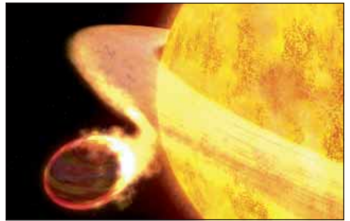
A csillagjához túl közel keringő „forró Jupiter” típusú bolygó anyaga folyamatosan párolog
