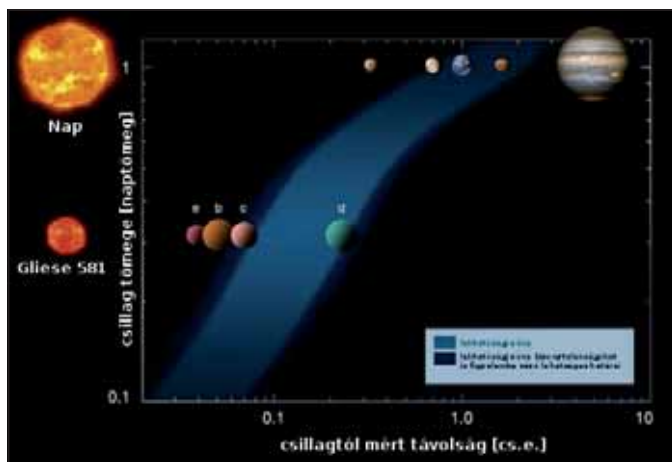
A lakhatósági zóna mérete a Naprendszerben és egy törpe csillag körül
