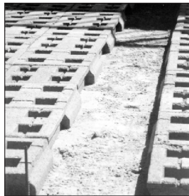
A MOBUR térkövek oldalkialakítása
