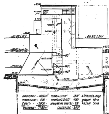
2. számú rajz. A békésszentandrasi duzzasztómű hosszmetérete.
