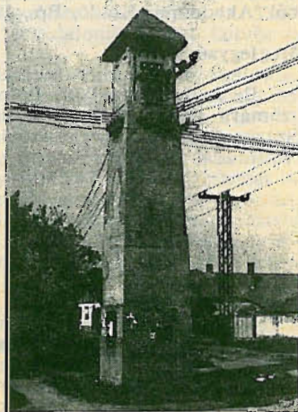
A tervezett, és egy ma is álló — használaton kívüli — transzformátorház
